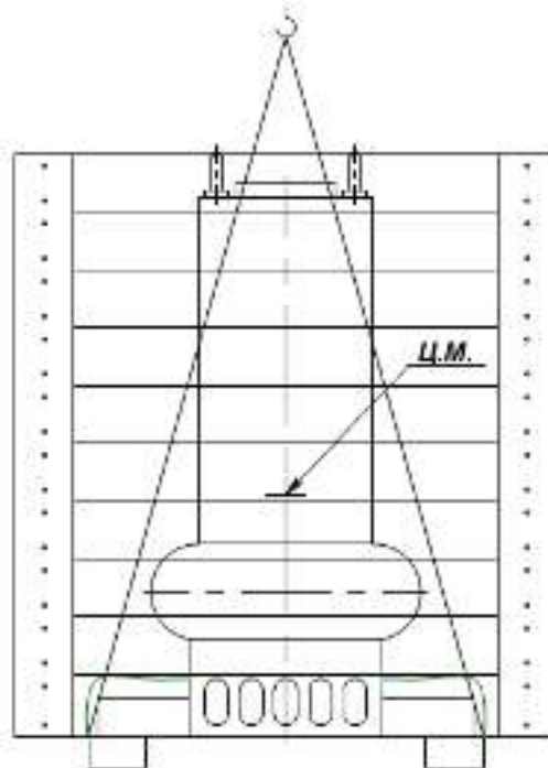
Рис. 1 Схема строповки насоса в таре
